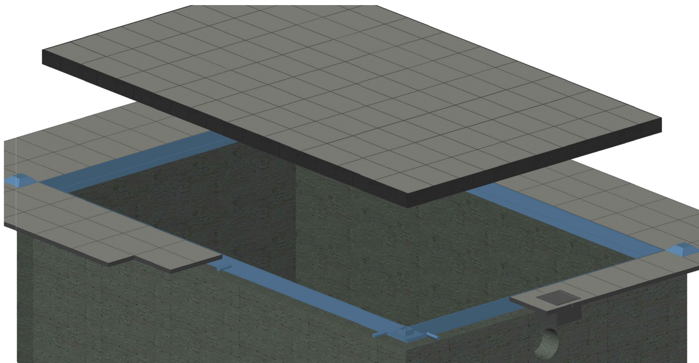
TETTO DI COPERTURA E CANALINA DI RACCOLTA ACQUA
