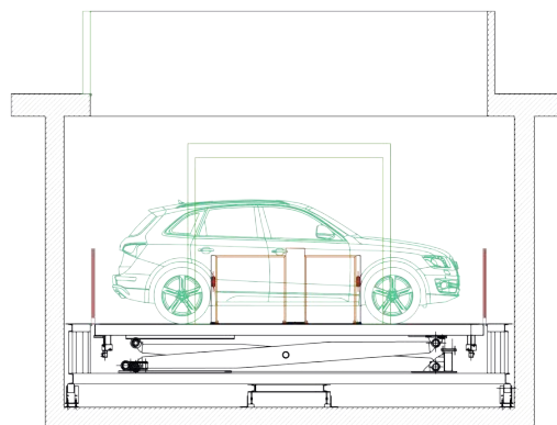
SEZ. A-A
