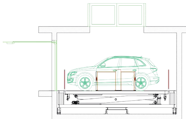
SEZ. B-B
