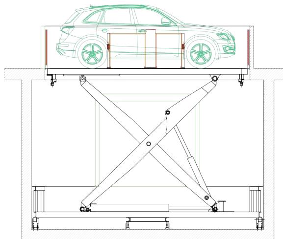
SEZ. A-A
